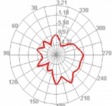
2500.000MHz E2
