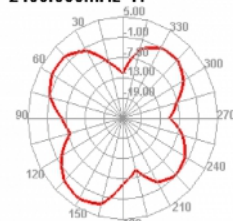
2450.000MHz
