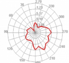
2400.000MHz E1
