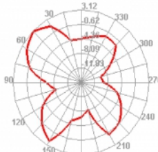
2400.000MHz
