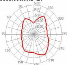
3800.000MHz E1
