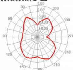
3800.000MHz E2
