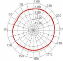
2500.000MHz H
