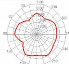
2450.000MHz E1
