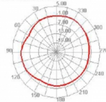
2450.000MHz H
