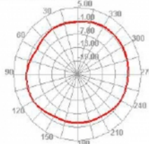
2500.000MHz H
