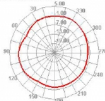
2450.000MHz H
